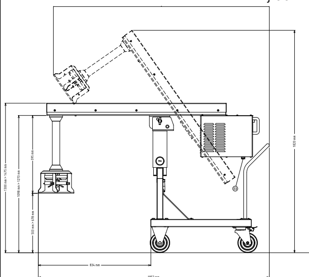
Zij aanzicht
